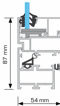
сечение окна
