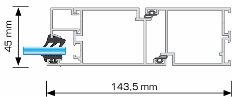
сечение двери
